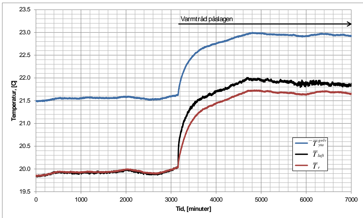
Figur 14 Lufttemperatur, golvttemperatur och motstrålande yttemperatur för försöket med lätt golvvärme.
