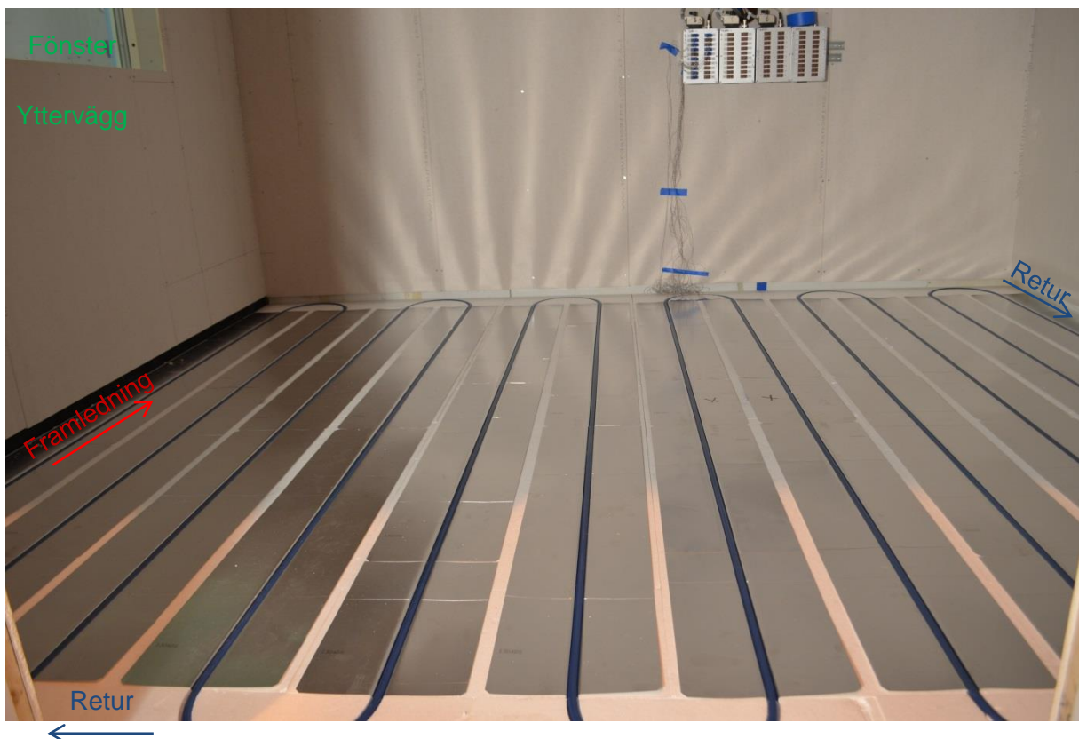
Figur 19 Lätt golvvärme med spårad EPS-isolering med värmefördelade aluminiumplåtar och PEX-rör. Bilden visar förläggningen av testrummets golvvärmeslinga. Pilarna indikerar vattnets flödesriktning i golvvärmeslingan.
