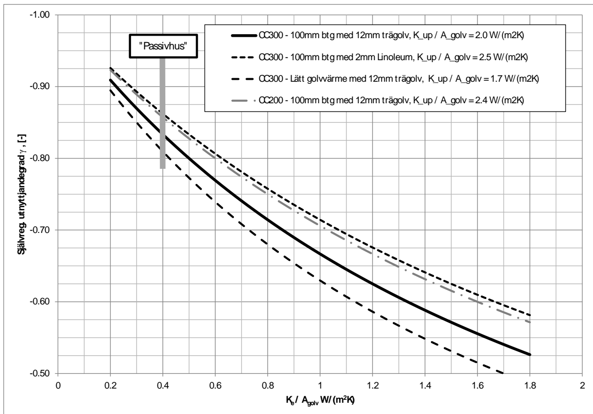
Figur 1 Exempel för utnyttjandegraden \gamma för varierande grad av värmeförluster. Beräknad värmeavgivning K_{up} med betongens värmeledningsförmåga ( \lambda=1.2 \text{ W/(mK)} ) och ytöverföringen ( \alpha_c + \alpha_r = 8 \text{ W/(m}^2\text{K)} ) i samtliga fall. Nivån för "passivhus" skall mer ses som en indikation än ett definitivt värde.
