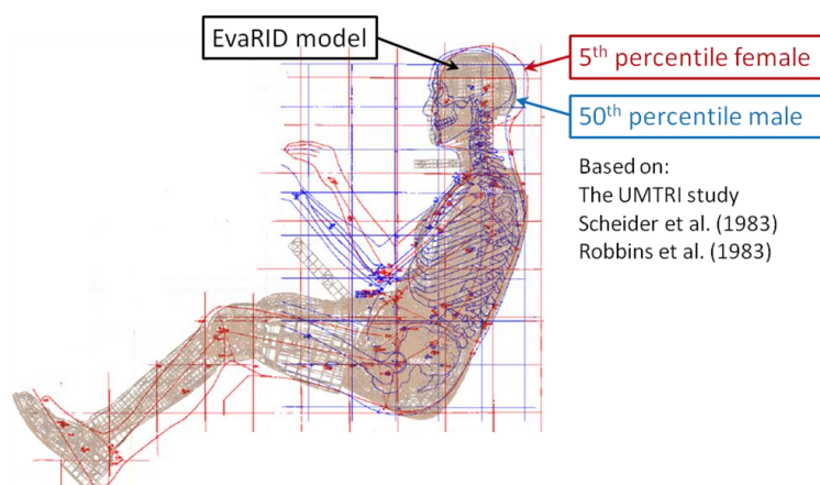
Figur 7. Jämförelser av en uppskalad 5-percentil kvinna (röda konturer), en nedskalad 50-percentil man (blå konturer) och en FE modell (EvaRID) som motsvarar BioRID50F-prototypen i storlek.
