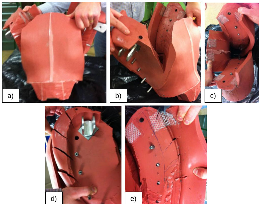
Figur 12. Djupa jack skars i gummitorson i syfte att minska dess styvhet. a) Frontvy. b) Sidoby (snett framifrån) c) Toppvy d) Sidvy (snett bakifrån) e) Innervy (bakre delen).
