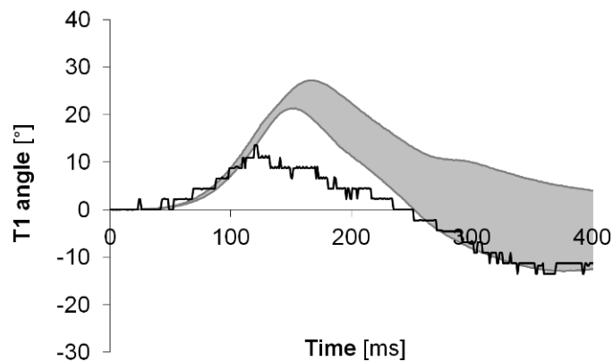
Figur 11. Överkroppens rotation hos den ursprungliga BioRID50F (heldragen svart linje) och kvinnliga volontärer (grå korridor).
