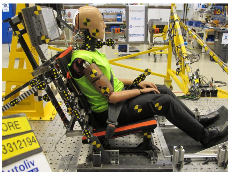
Figur 16. Provuppställning – dynamiska prov.
