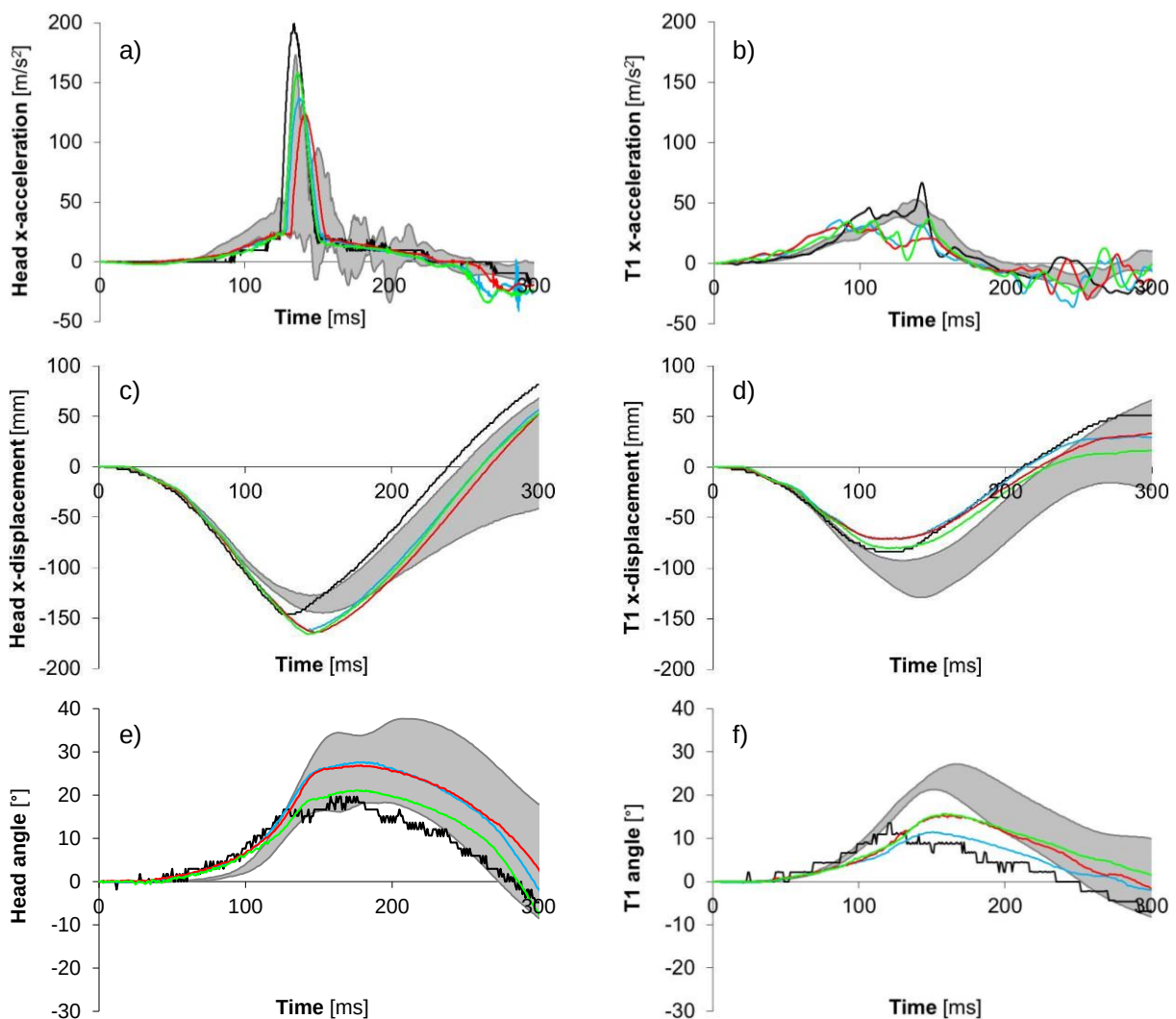
Figur 19. Släddprovning (upphinnandekollisioner) med volontärer (grå korridorer), BioRID 50F_V1 (svart linje) och BioRID 50F_V2 (T-13312194 = blå; T-13312195 = röd; T-13312196 = grön).
