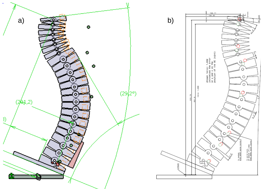
Figur 9. a) CAD-modell av BioRID 50F:s ryggrad, samt ledpunkter (gröna punkter) för den 5-percentila kvinnan enligt UMTRI-studien (Schneider et al. 1983). b) Slutlig ryggkurvatur för BioRID 50F_V2, samt uppskalade ledpunkter (röda cirklar).
