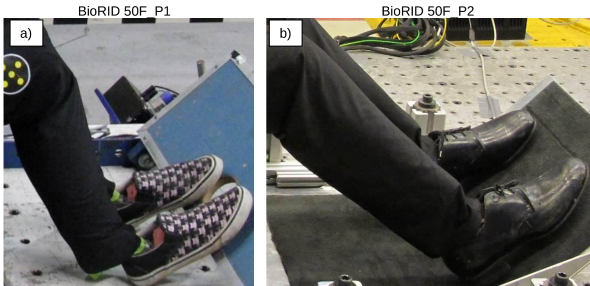
Figur 3. a) Underben på BioRID 50F_P1 (nerskalade delar från BioRID 50M plus enkel ankel- och fotkonstruktion). b) Underarmar på BioRID 50F_P2 (modifierade delar från Hybrid III 5F).
