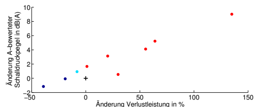
Abbildung 1: Ergebnisse Parameterstudie für reifenunabhängige Parameter. + Ausgangskonfiguration. Farben identifizieren unterschiedliche Kombinationen von Ab-/Zunahme für Rollgeräusch/-widerstand.
