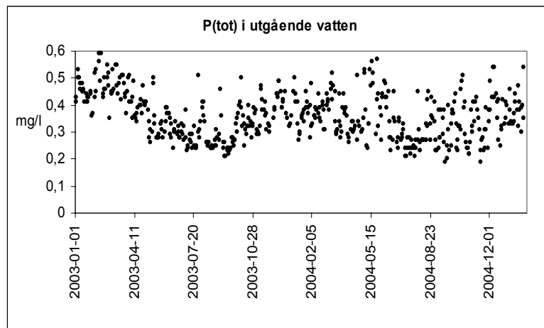
Diagram 1. Totalfosfor i utgående vatten (mg P/l); dygnsmedel
