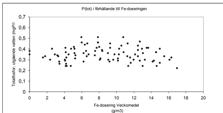
Diagram 5. Förhållandet mellan järndosering och P (tot.) ut ; veckomedel under tiden 2003-01-01 till 2004-09-20
