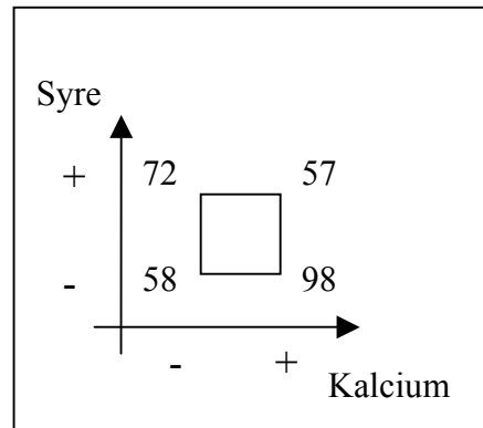
Bild 20. Interaktion Syre Kalcium Omgång 3, Järn
