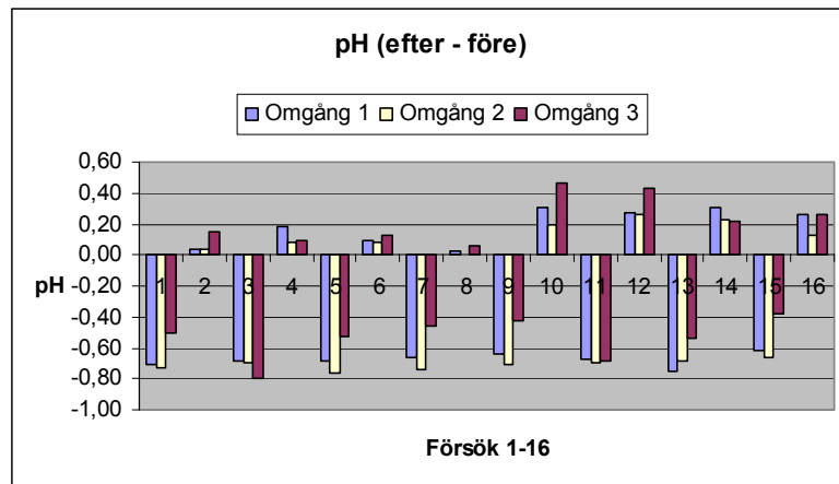
Diagram 25. pH förändringar vid försök 1-16.
