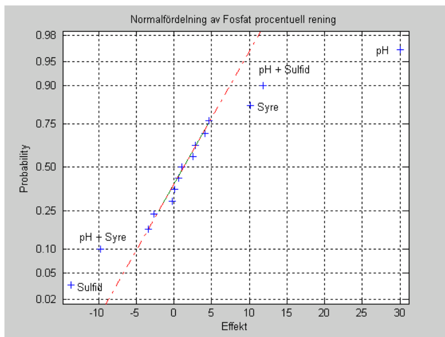
Diagram 14. Normalfördelningsplot av effekterna vid den procentuella reningen av fosfat
