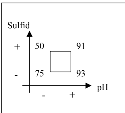
Bild 23. Interaktion fosfat, pH + Sulfid
