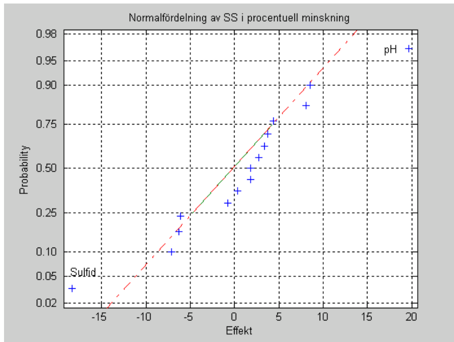
Diagram 12. Normalfördelningsplot av effekterna vid den procentuella minskningen av SS.
