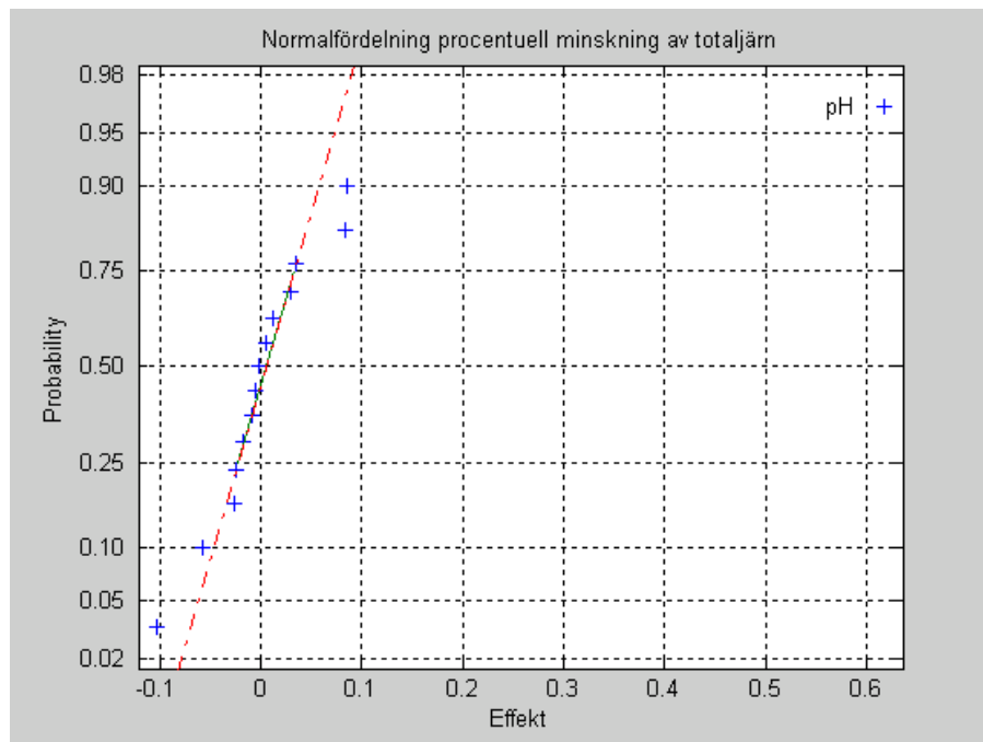
Diagram 19. Normalfördelningsplot av effekterna vid den procentuella minskningen av totaljärn
