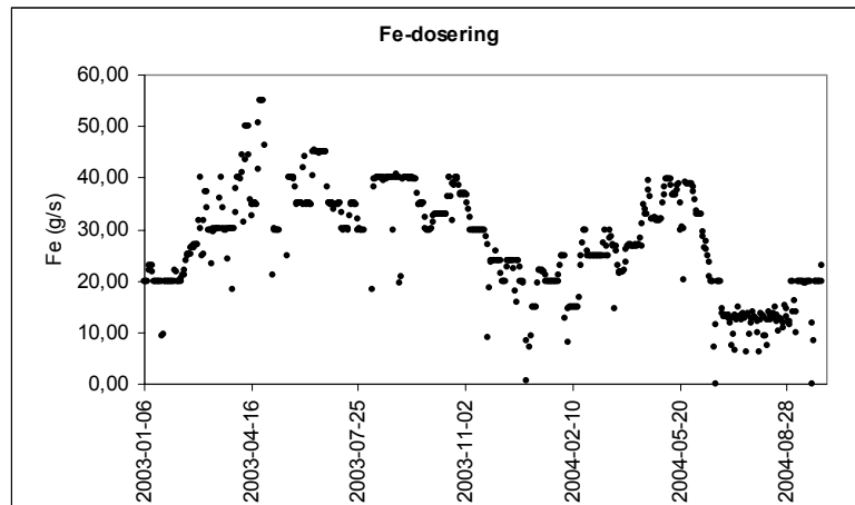
Diagram 4. Dosering av järn (g/s); dygnsmedelvärde under tiden 2003-01-01 till 2004-09-20
