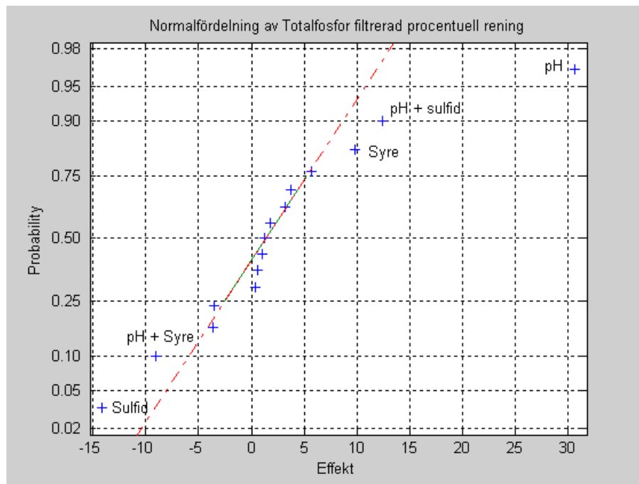
Diagram 16. Normalfördelningsplot av effekterna vid den procentuella reningen av totalfosfor
