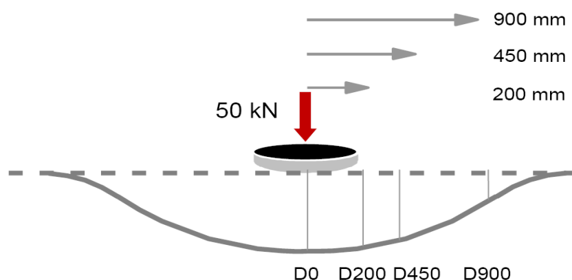
Figur 2.9 Sjunctratt FWD (Vägverket 1998)
