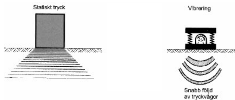
Figur 2.4 Schematisk figur över olika packningsmetoder (Forssblad, 2000)
