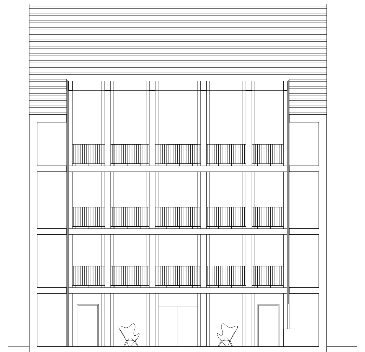
SEKTION B-B SKALA 1:100
