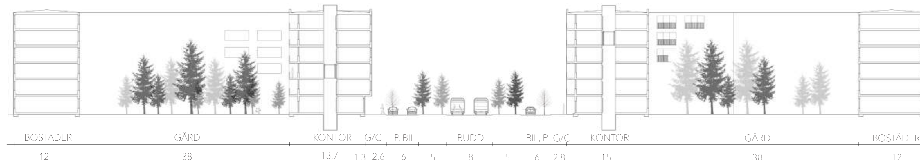
SEKTION B-B SKALA 1:400
