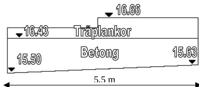
Figur 14: Tvärsnitt A-A, tvärsektion av Danagatans bräddavlopp
