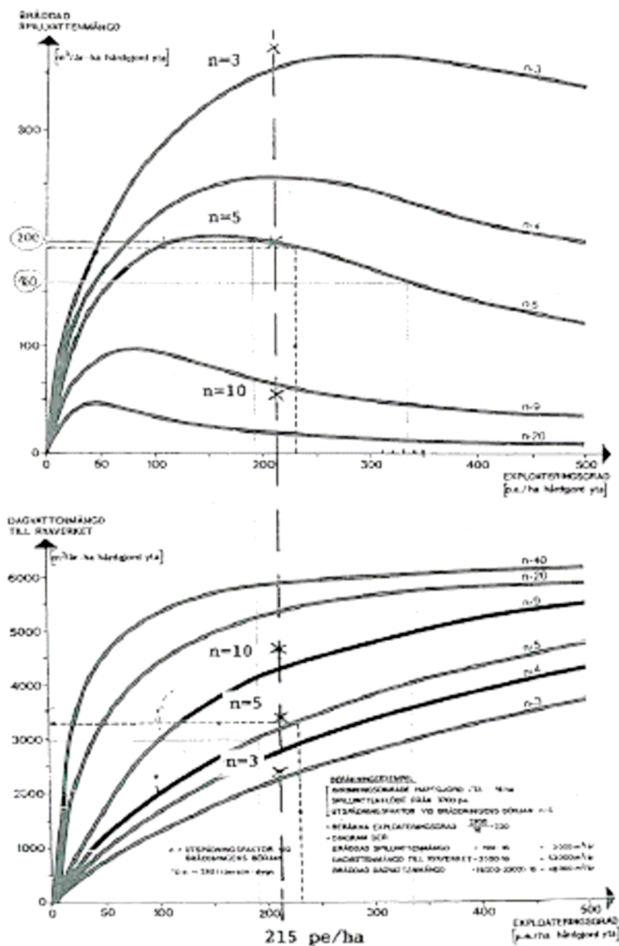
Bräddad spillvattenmängd och dagvattenbelastning på Ryaverket från kombinerat system - beräkningsdiagram
