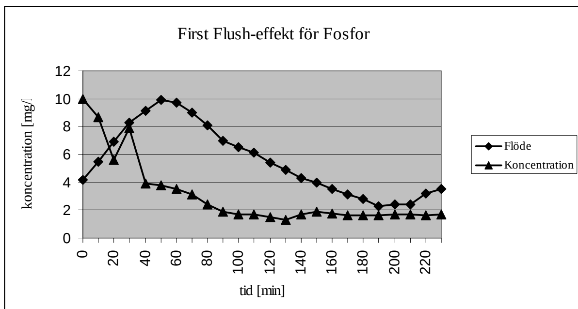
Figur 2: Variationen i fosforkoncentrationen under ett bräddtillfälle 940629 i ett bräddavlopp i Bellevue, Göteborg. Bräddtillfället har föregåtts av sju torrdrygn.
