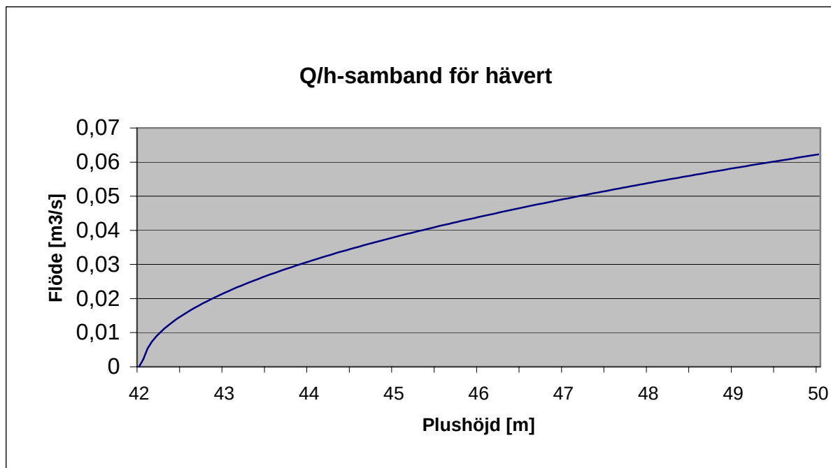
Figur 21: Q/h-samband för Molnvädersgatus hävert
