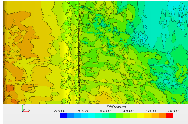
(a) LES
