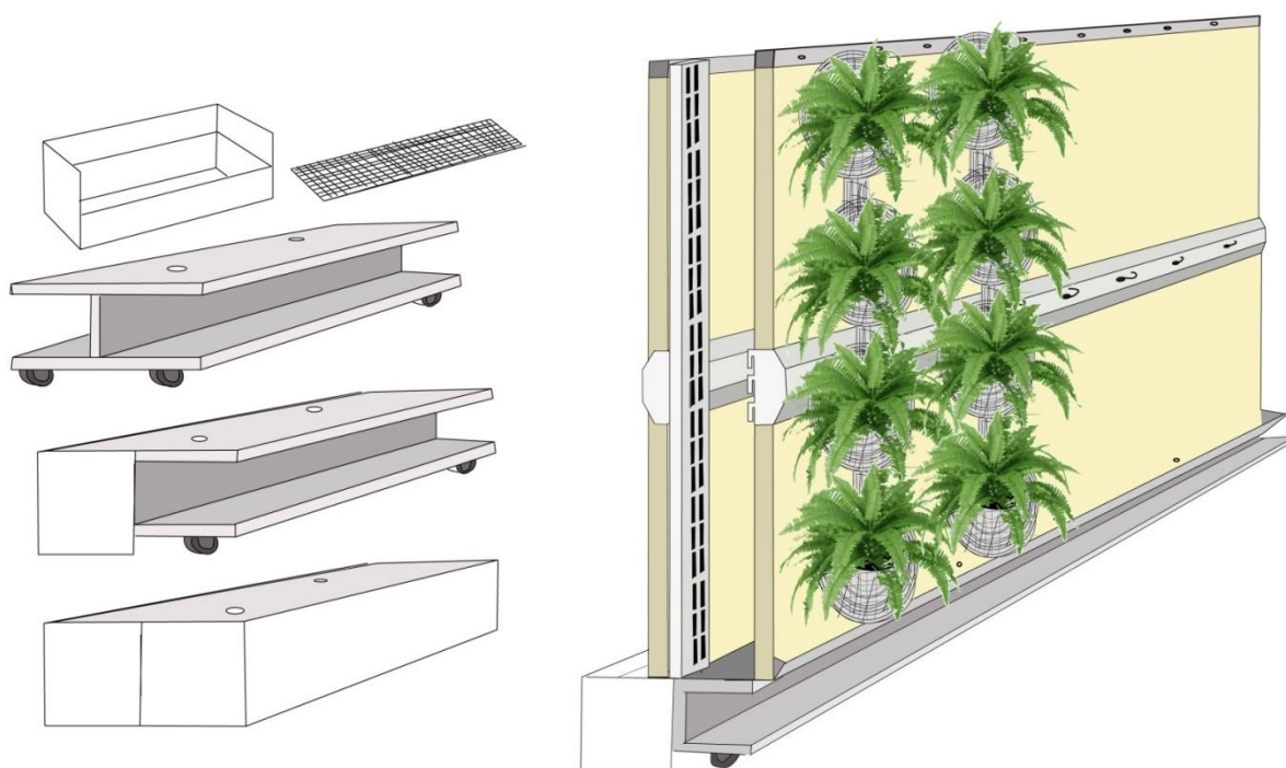
Figur 6.3 - Den mobila lösningen med vattenuppsamling samt stomme
