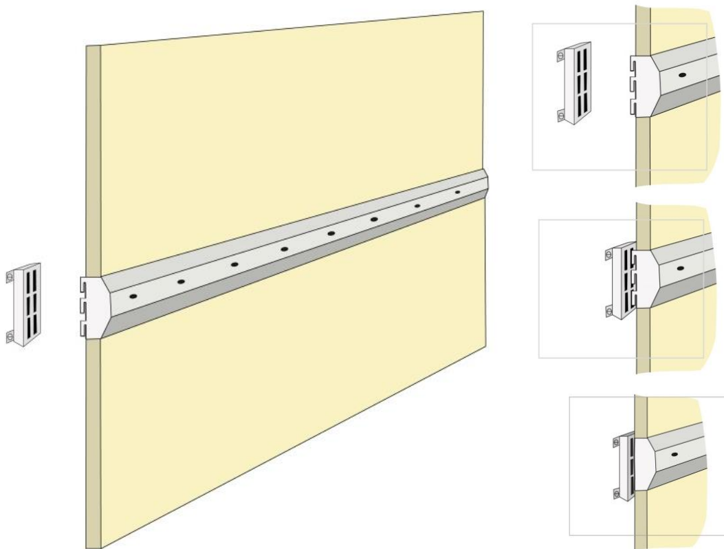
Figur 6.1 - Stomme av Diaboard, med sammanfogning och väggfäste
