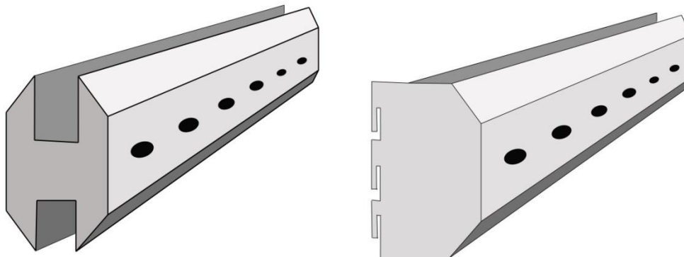
Figur 6.2 - "I-balken" som fäster ihop Diaboard-skivorna
