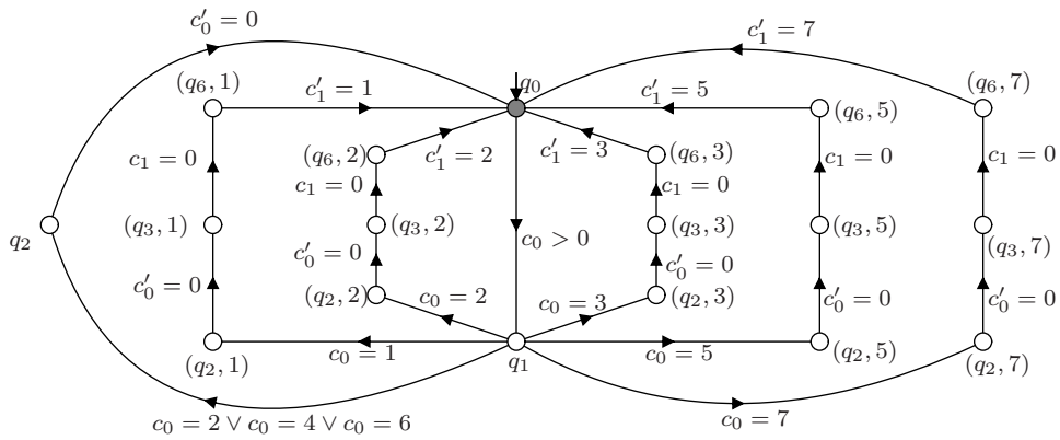
U(S_1)
