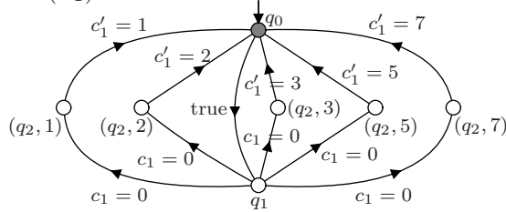
U(S_1)
